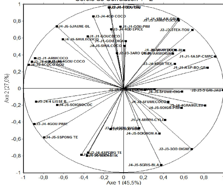
A.C.P. horizontale des moyennes (Pondération de STATIS) : profil libre comparatif Cercle de Corrélation 1 - 2
