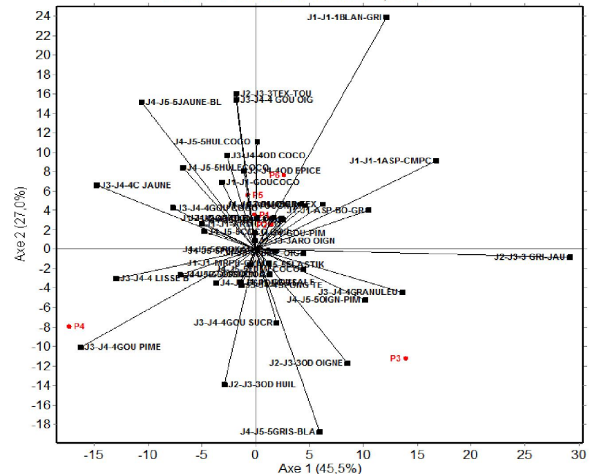
A.C.P. horizontale des moyennes (Pondération de STATIS) : profil libre comparatif Plan 1 - 2 Constante BiPlot : 54,23299
